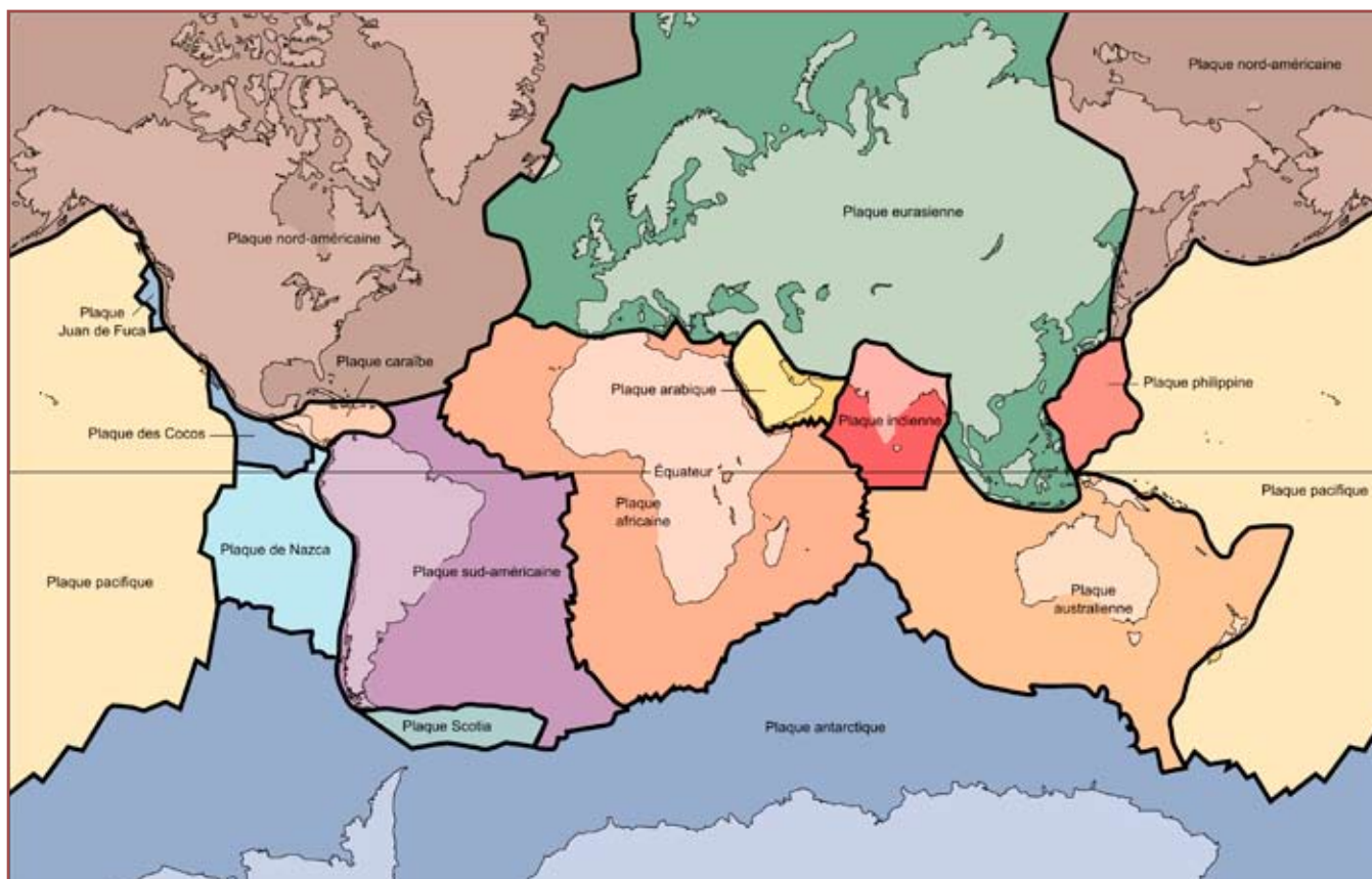
Figure 4 : les principales plaques et leurs limites (d'après un document de l'U.S. Geological Survey, 2001).
