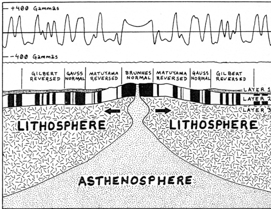
Figure 5 : formation des anomalies magnétiques au niveau d'une dorsale médio-océanique. Les parties noires et blanches représentent des roches dont la polarité magnétique est alternativement normale (noir) et inverse (blanc). Les différentes époques magnétiques sont désignées par les noms de géomagnéticiens célèbres (Brunhes, Matuyama, Gauss, Gilbert). L'échelle d'inversion de polarité (appelée magnétostratigraphie) est symétrique de part et d'autre de la dorsale comme le montre clairement le profil magnétique (l'intensité du champ magnétique est exprimée en Gamma, avec 1 Gamma = 1 nanoTesla).
