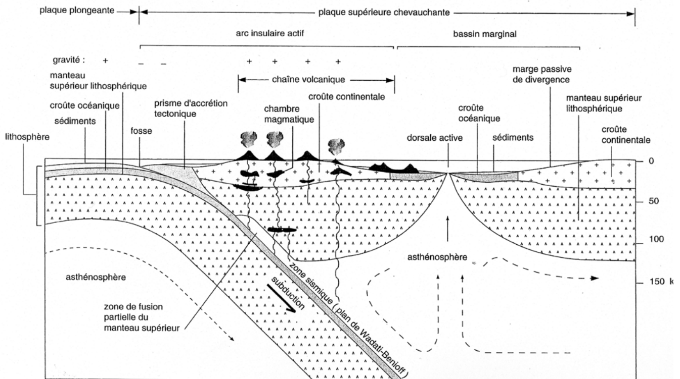
Figure 6 : coupe schématique d'une zone de subduction (d'après Juteau et Maury, 2005).
