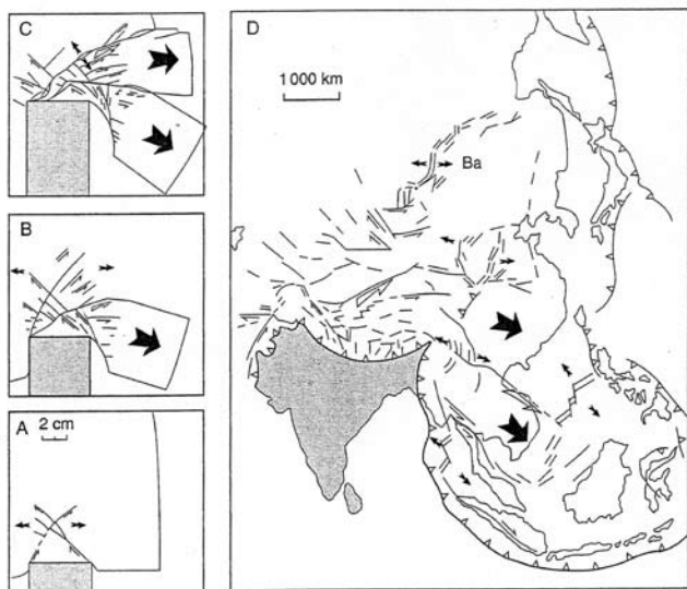
Figure 7 : modèle de poinçonnement de l'Asie par le sous-continent indien (d'après le modèle de Tapponier et al, 1986, repris par Boillot et al, 2008).
