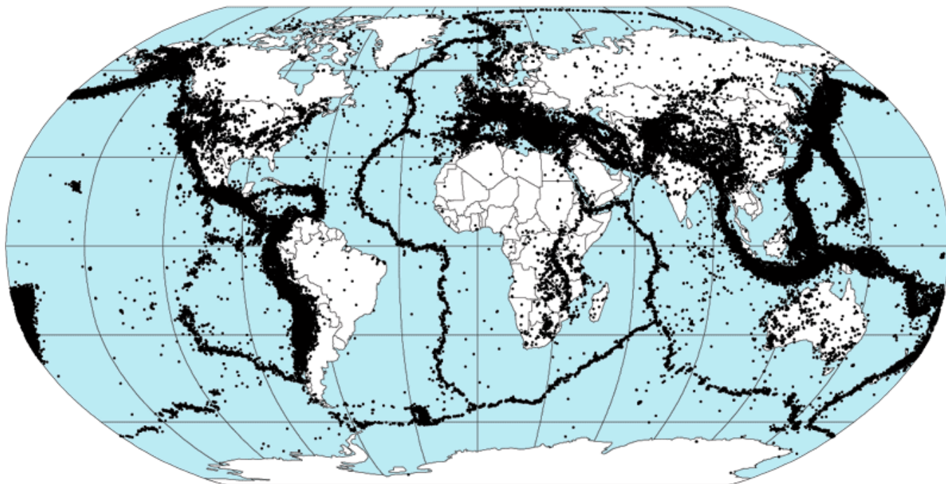
Figure 3 : localisation des épicentres des séismes. La répartition de ces séismes le long de ceintures sismiques longues et étroites indique la limite des plaques actuelles (Boillot et al, 2008, d'après Gordon et Stern, 1992).
