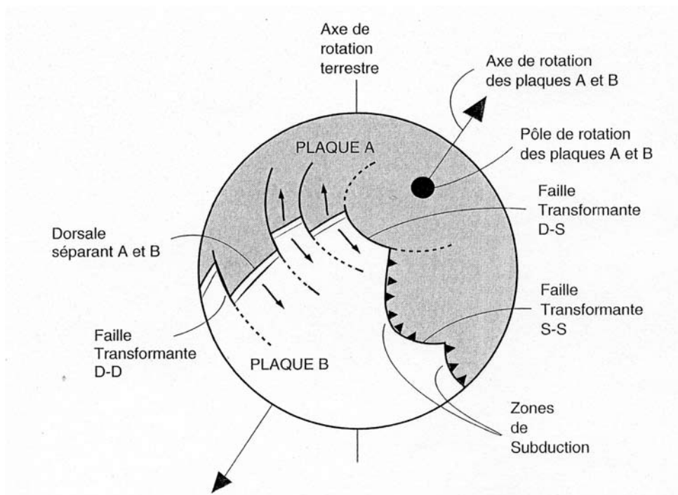
Figure 8 : rotation de deux plaques A et B à la surface de la Terre. Les failles transformantes sont des petits cercles centrés sur l'axe eulérien de rotation des plaques. Elles raccordent soit une dorsale à une zone de subduction (faille D-S), soit deux zones de subduction (faille S-S). (d'après Allègre, 1984).
