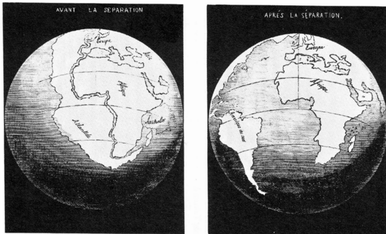
Figure 1 : premier modèle de mobilité des masses continentales publié dans « La création et ses mystères dévoilés » d'Antonio Snider-Pelligrini (1858). Reconstitution de la position de l'Amérique du Sud et de l'Afrique, avant et après la séparation entre ces deux masses continentales.
